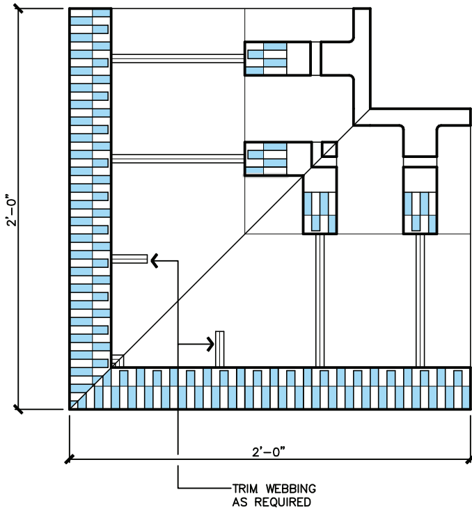
① TOP VIEW SCALE: 1 1/2" = 1'-0"
