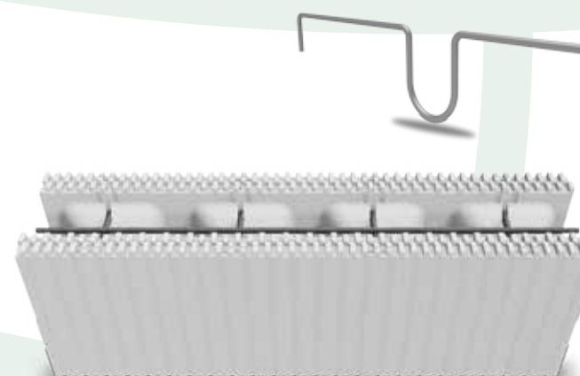
GLOBALBLOCK USANDO PEDAZOS DE BARRAS DE REFUERZO OPCIONALES.
