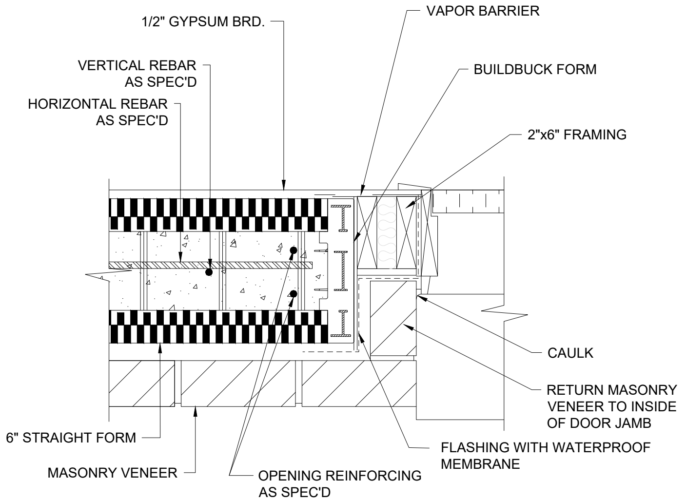
1 DOOR JAMB DETAIL 6 INCH
